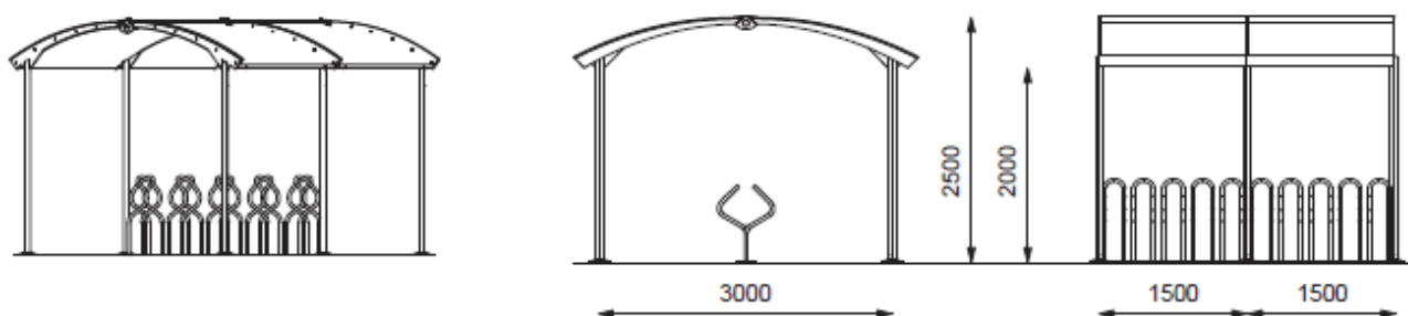
PUBLICUS ® dobbelt sykkelskur
