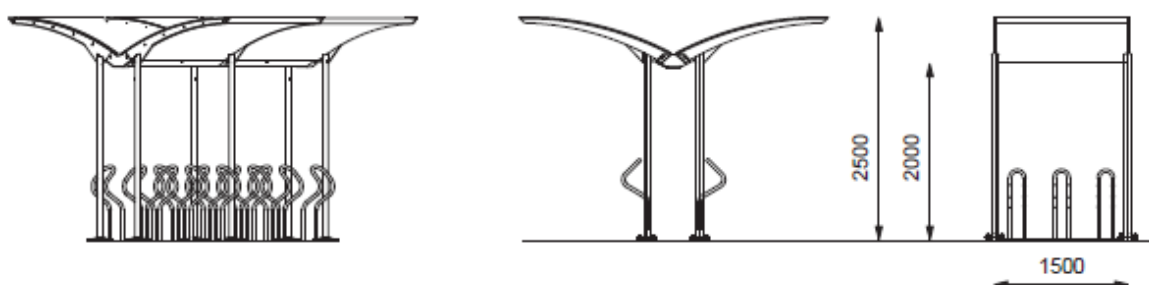
PUBLICUS ® sykkelskur - måkevinge
